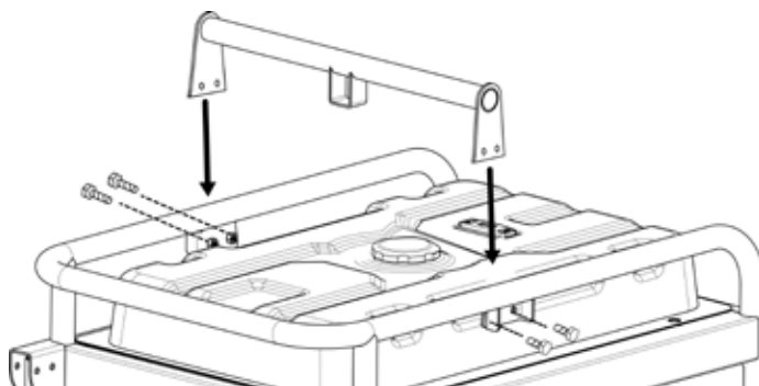
Figure 2 - Installation du support d'élévation
