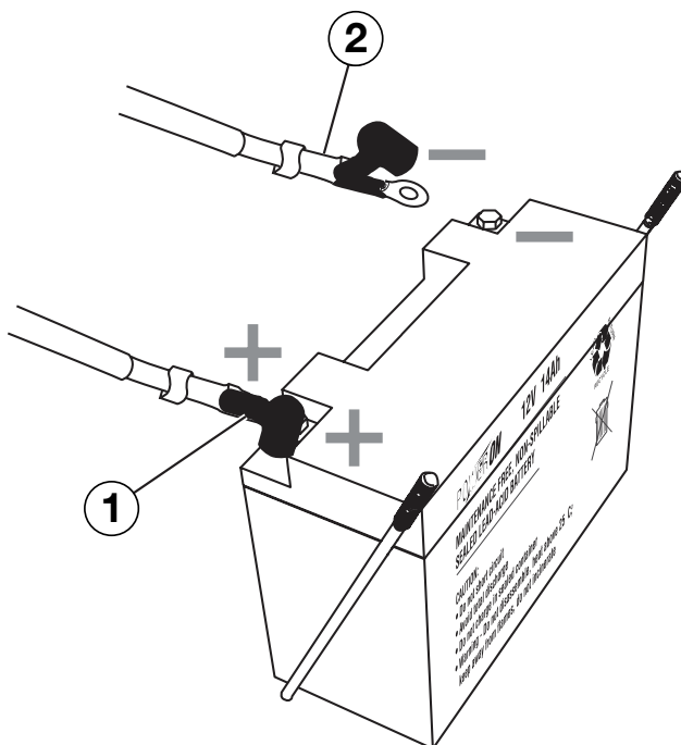
Figura 4 - Conecte la batería 1 - Cable positivo (+) de la batería (rojo) 2 - Cable de batería negativo (-) (negro)
