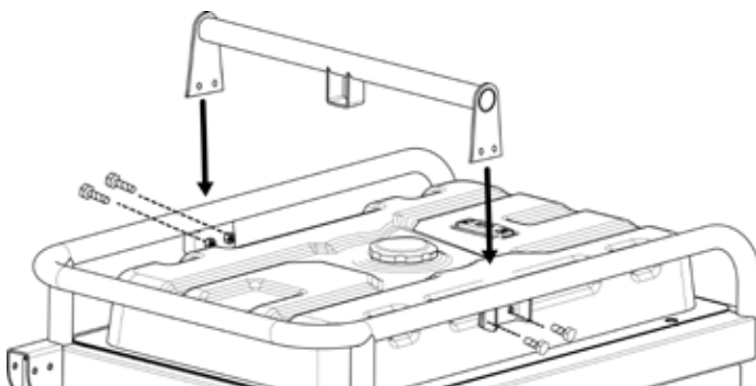
Figura 2 - Instale el soporte de elevación
