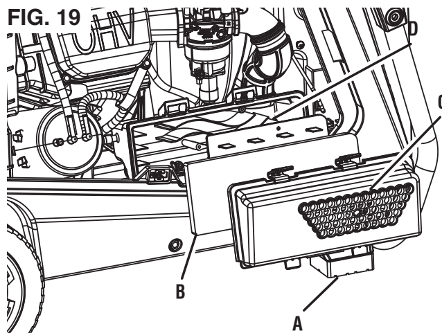
FIG. 19 A - Cubierta del filtro de aire B - Filtro de aire C - Lengüeta D - Caja del filtro de aire
