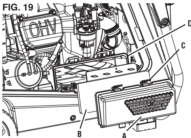
FIG. 19 A - Couvercle du filtre à air B - Filtre à air C - Languette D - Boîte de filtre à air
