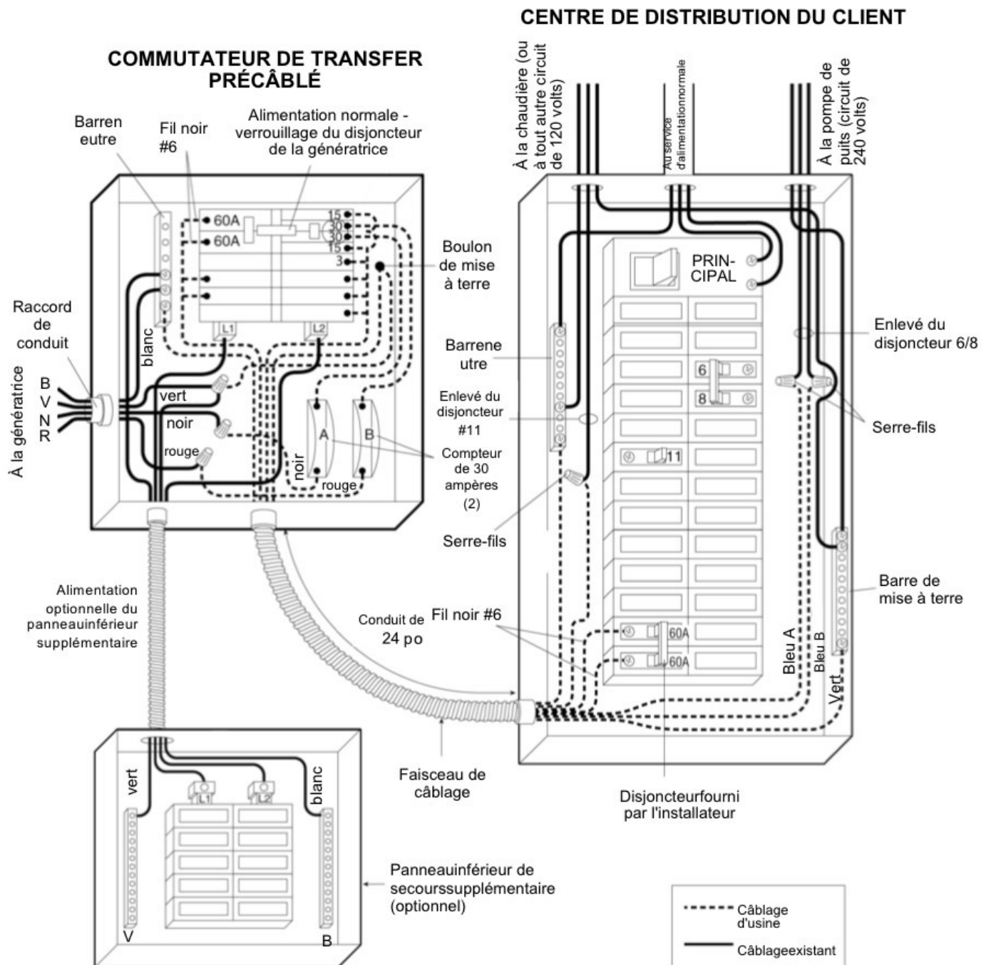
Figure 2: DIAGRAMME DE CÂBLAGE
