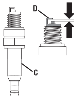
A - Bougie B - Soufflet de bougie d'allumage C - Isolant D - Électrode
