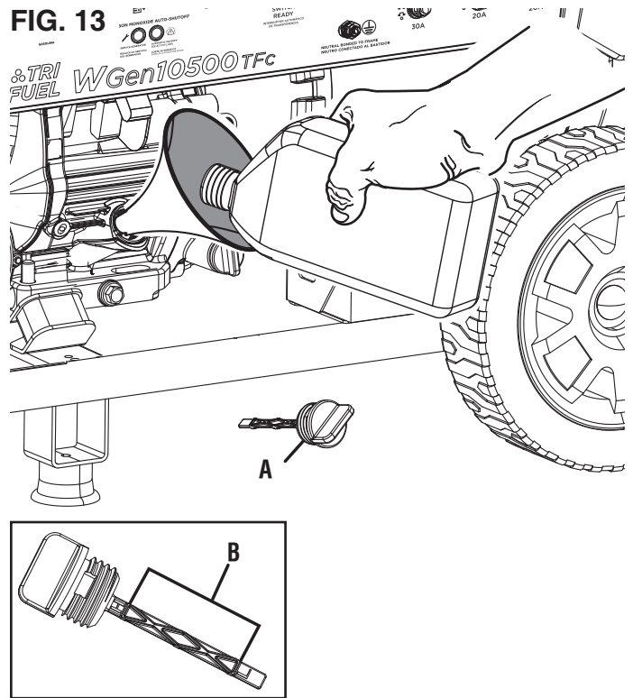
A - Jauge d'huile B - Plage de fonctionnement sécuritaire
