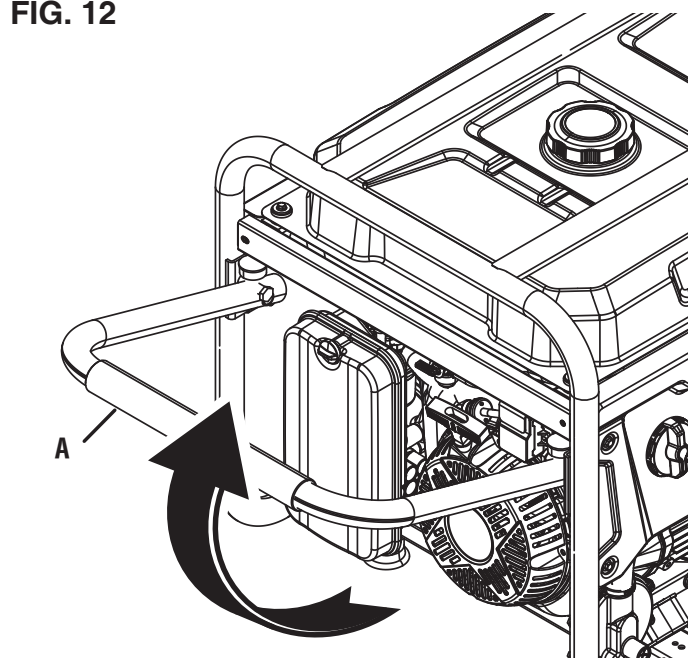
A - Poignée
