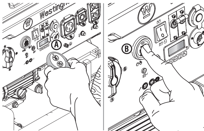
A - Porte-clés B - Bouton de démarrage/arrêt du moteur
